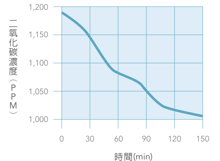
實測植生牆沉降二氧化碳曲線
